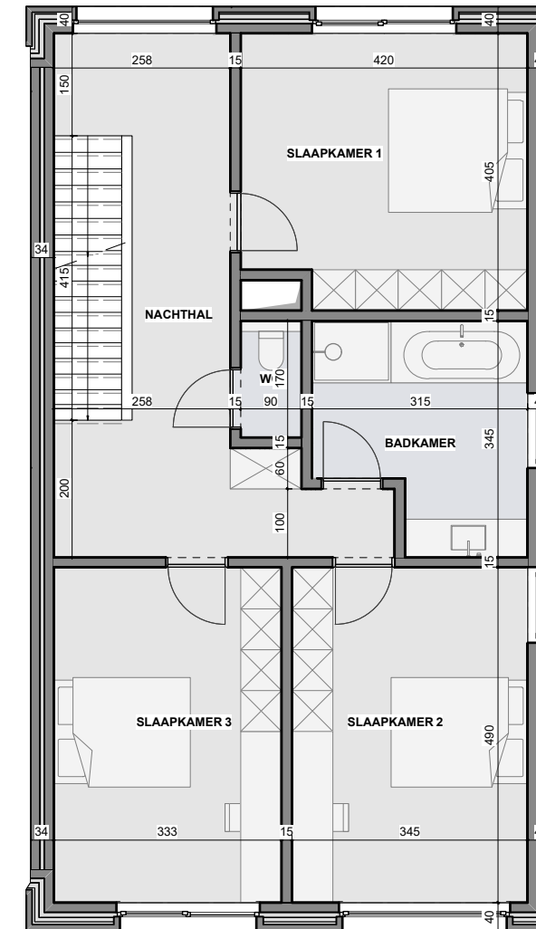
grondplan +01
