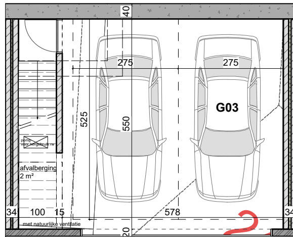
grondplan garage -01
